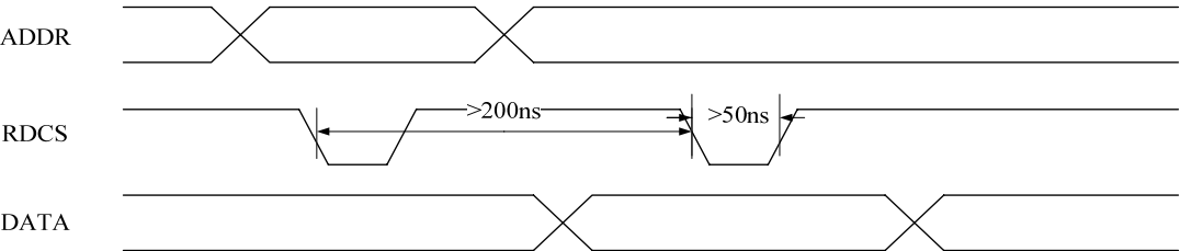
读时序
