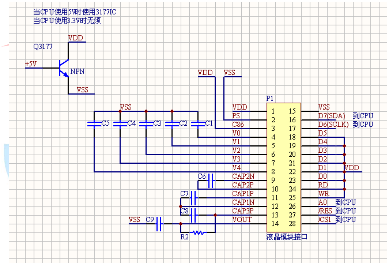
图 9. 串行接口
