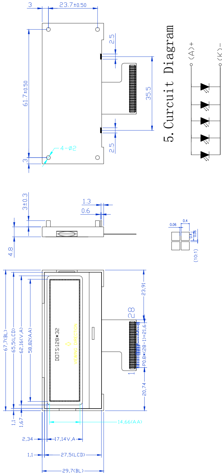
图 1. 外形尺寸
