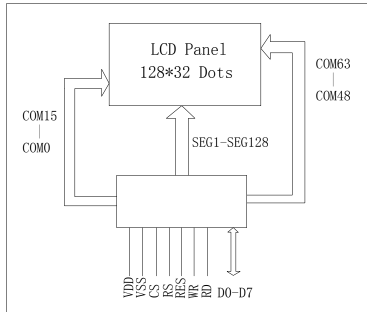
图 2 X12832A-3G 图像点阵型液晶模块的电路框图
