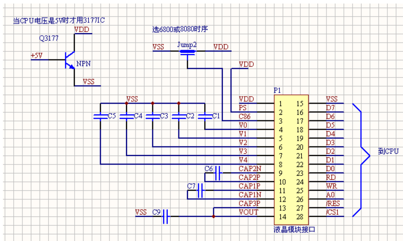
图 8. 并行接口
